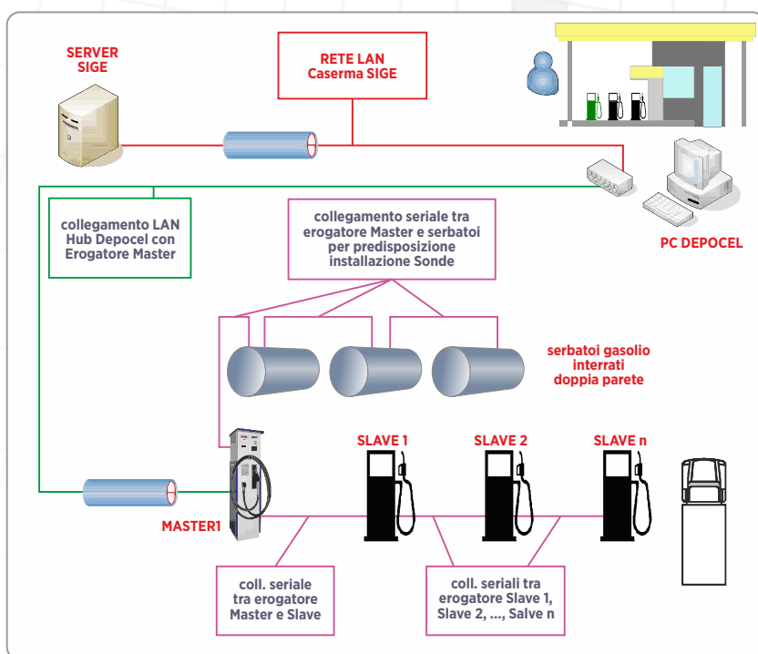
Easy Fuel®: Schema informatizzazione DepoCel
